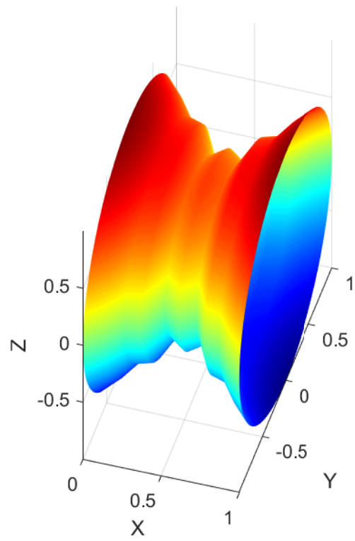
Sólido de revolución ( n=10 , t_k=0.15 )
